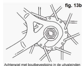
Achterwiel met boutbevestiging in de uitvaleinden
